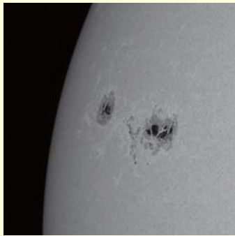
太陽黒点
